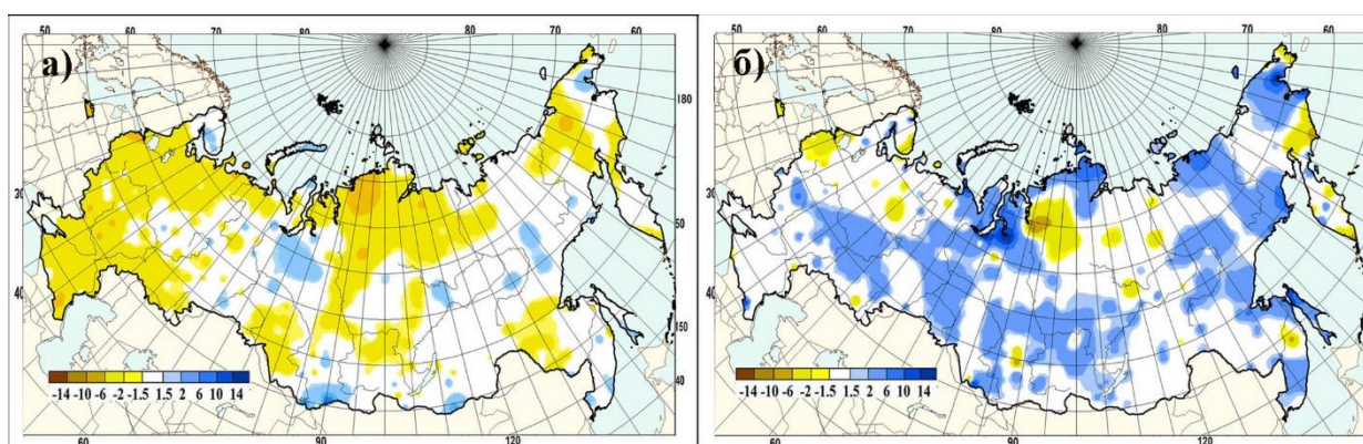
Рисунок 3.4 – а) Коэффициенты линейного тренда (см/10лет) в рядах максимальной за зимний период высоты снежного покрова. б) Коэффициенты линейного тренда (дни/10лет) в рядах числа дней со степенью покрытия окрестностей станции снегом более 50%. 1976-2023 гг.
