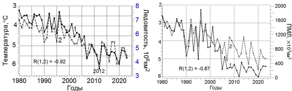
Рисунок 6.3 – Площадь, занятая морским льдом в сентябре (1), и летняя температура воздуха (2) на акватории Северного Ледовитого океана (а) и морей Северного морского пути (б) в 1980–2023 гг.
