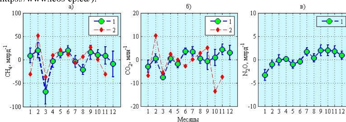
Рисунок 16.5 – Разность среднемесячных концентраций \text{CH}_4 (а), \text{CO}_2 (б), \text{N}_2\text{O} (в) в приземном слое атмосферы в 2023 г. относительно 2022 г. 1 – Обнинск, 2 – Карлсруэ
