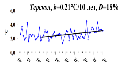
Рисунок 1.7 – Ход среднегодовых температур на метеорологических станциях с линейным трендом за период 1976-2022 гг.; b – значение углового коэффициента линейного тренда, °C/10 лет; D (%) – вклад тренда в суммарную дисперсию
