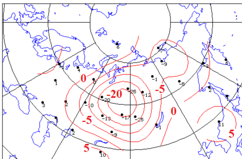
Рисунок 18.1 – Поле отклонений значений ОСО от средних многолетних значений 6 июня 2023 г., (%)
