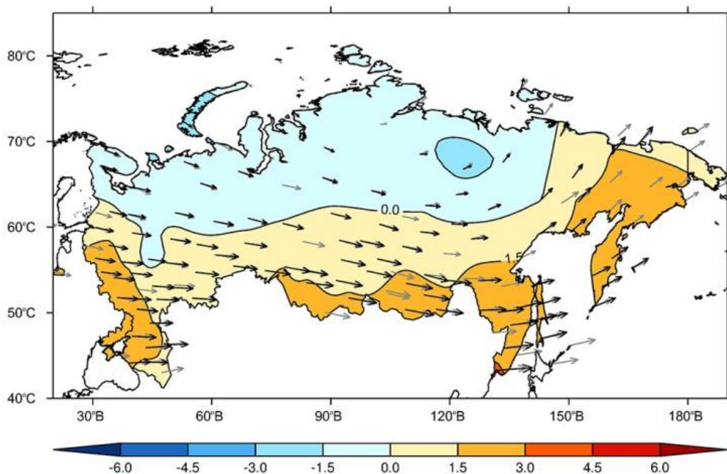
Рисунок 15.3 – Аномалии скорости ветра в 2023 г. в нижней стратосфере. Черные стрелки указывают среднее направление ветра в 2023 г., серые – за период 1985-2014 гг.
