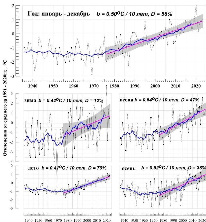
Рисунок 1.1 – Средние годовые (вверху) и сезонные аномалии температуры приземного воздуха (°C), осредненные по территории России, 1936-2023 гг.
