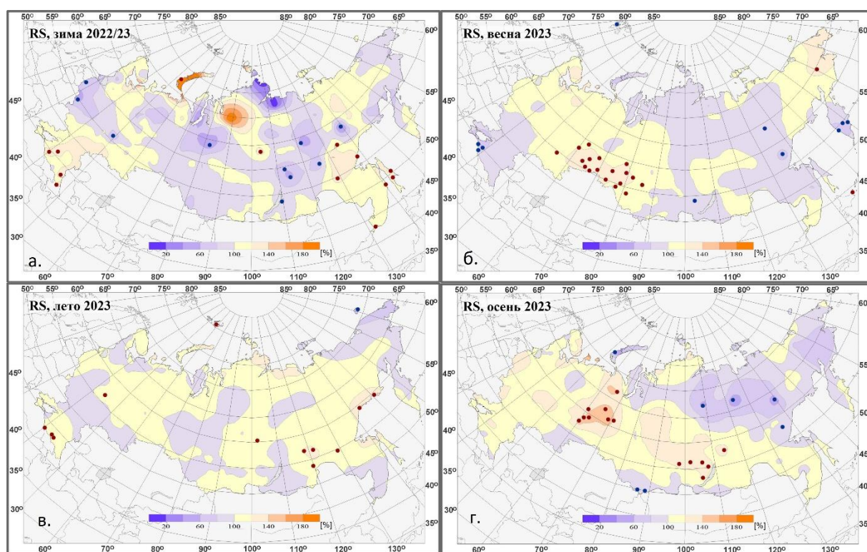
Рисунок 12.2 – Пространственное распределение относительных аномалий сезонной продолжительности солнечного сияния (RS, %) на территории РФ в 2023 г. Кружками синего цвета показано местоположение станций с экстремумами ниже 5-го процентиля, коричневого цвета – выше 95-го процентиля
