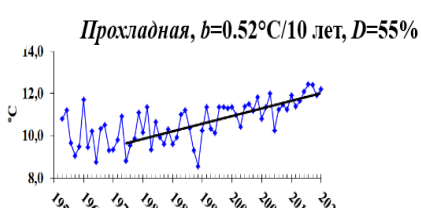
Рисунок 1.7 – Ход среднегодовых температур на метеорологических станциях с линейным трендом за период 1976-2022 гг.; b – значение углового коэффициента линейного тренда, °C/10 лет; D (%) – вклад тренда в суммарную дисперсию
