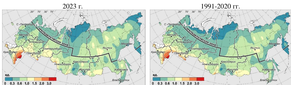
Рисунок 8.2 – Индекс сухости М.И. Будко за 2023 г. и средние значения за 1991–2020 гг.
