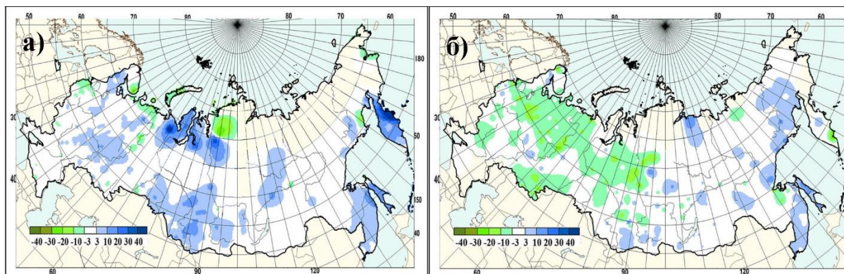
Рисунок 3.5 – Коэффициенты линейного тренда (мм/10лет) в рядах запаса воды в снеге за зимний период в поле (а) и в лесу (б). 1976-2023 гг.
