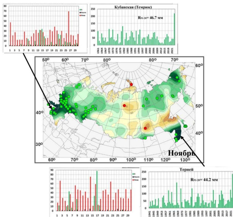
Рисунок 2.4 – Аномалии осадков в ноябре 2023 г. На врезках ряды месячных и суточных сумм осадков на метеорологических станциях Кубанская и Терней в зонах значительного переувлажнения
