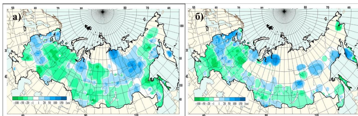
Рисунок 3.3 – Аномалии максимального запаса воды в снеге (мм) зимой 2020-2023 гг. (от среднемноголетних значений за период 1971-2000 гг.) в поле (а) и в лесу (б)
