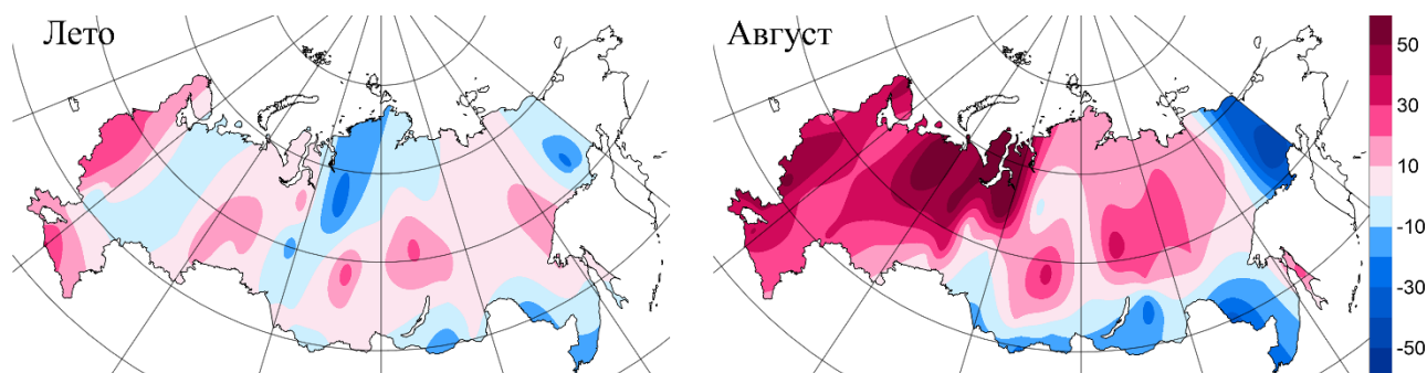
Рисунок 10.6 – Аномалии (в процентах от среднего за 1961-1990 гг.) сезонных и месячных (август) сумм прямой солнечной радиации. Лето 2023 г.
