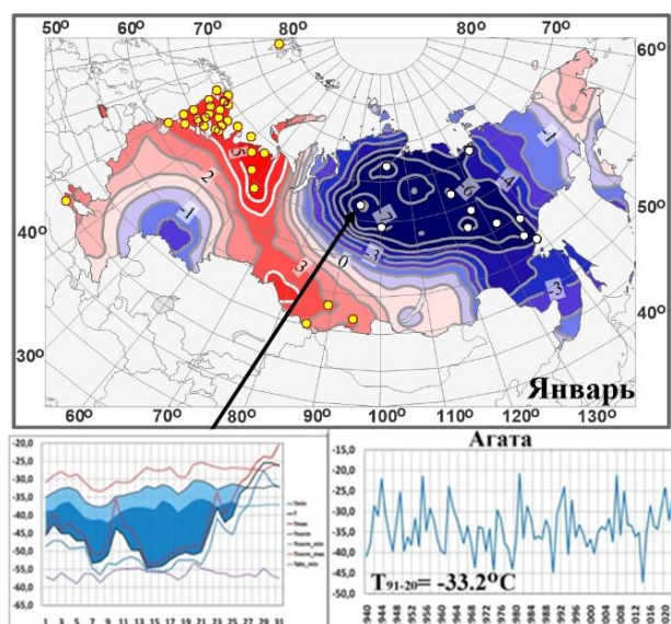
Рисунок 1.3 – Аномалии температуры приземного воздуха на территории России в январе 2023. На врезках ряды среднемесячной январской температуры воздуха и среднесуточной температуры воздуха в январе 2023 года на метеорологической станции Агата в очаге отрицательных температурных аномалий
