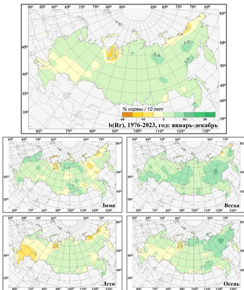
Рисунок 2.5 – Пространственные распределения локальных коэффициентов линейного тренда годовых и сезонных сумм атмосферных осадков за 1976-2023 гг. на территории России (% /10 лет)
