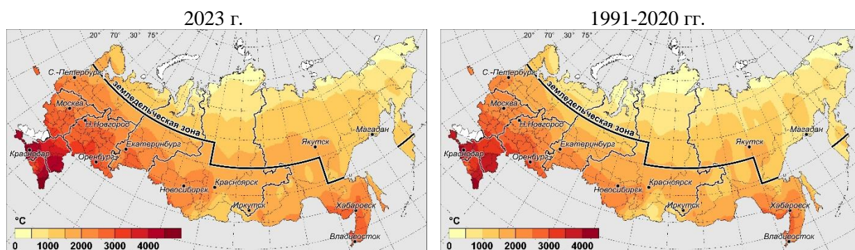
Рисунок 8.1 – Сумма температур выше 10^{\circ}\text{C} ( ^{\circ}\text{C} ) за 2023 г. и средние значения за 1991–2020 гг.
