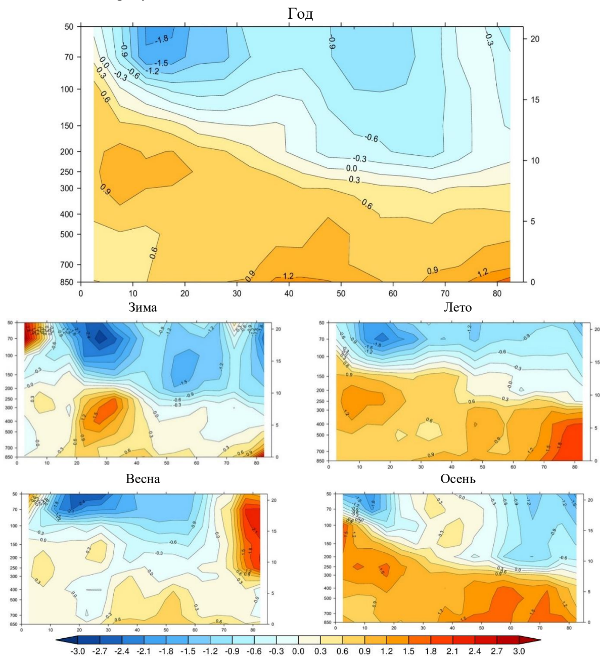
Рисунок 13.1 – Вертикально-широтная структура годовых и сезонных аномалий температуры свободной атмосферы в 2023 г. Горизонтальная ось – широты, левая вертикальная ось – давление на стандартных изобарических поверхностях, правая вертикальная ось – высоты над уровнем моря, в км
