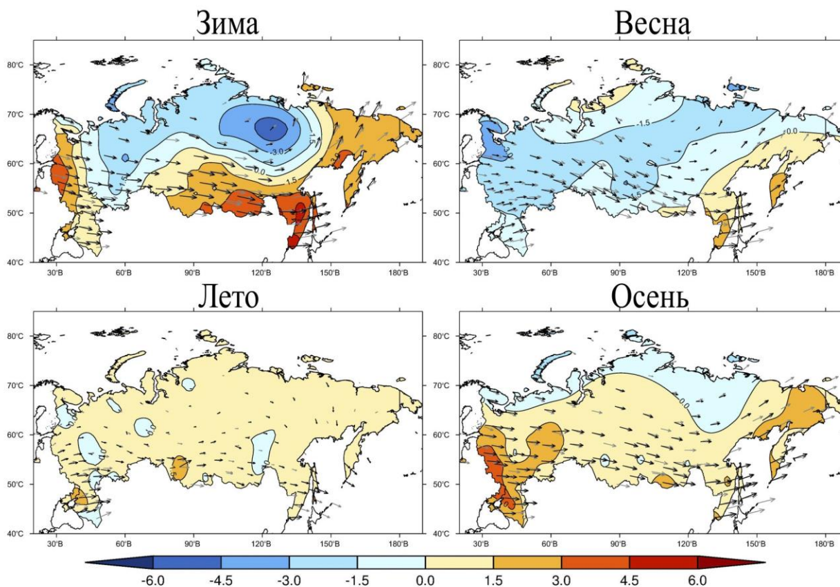
Рисунок 15.4 – Аномалии скорости ветра для отдельных сезонов (зима 2022/2023 гг., весна, лето и осень 2023 г.) в нижней стратосфере.
