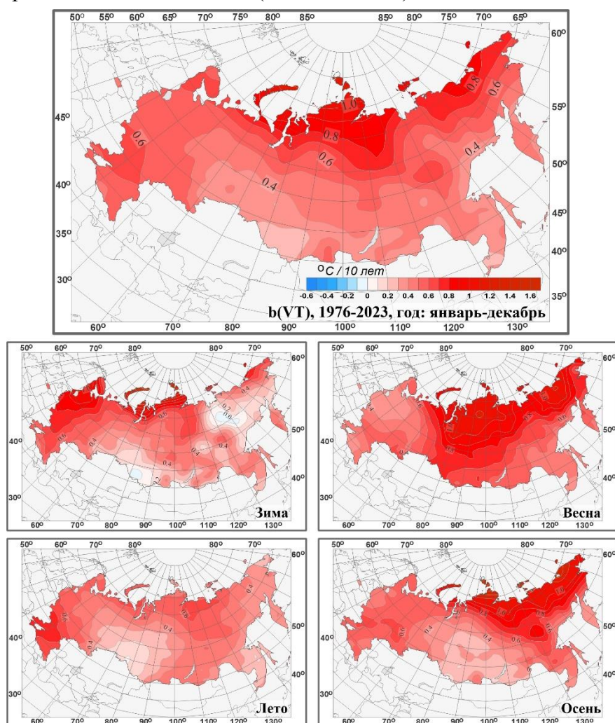
Рисунок 1.6 – Коэффициент линейного тренда среднегодовой и средних сезонных значений температуры приземного воздуха на территории России за период 1976-2023 гг. (°C/10 лет)
