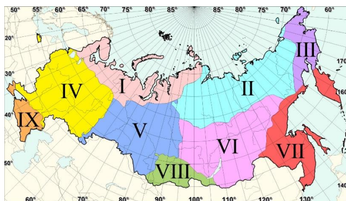
Рисунок 3 – Квази-однородные климатические регионы (используются в разделах: «Снежный покров», «Продолжительность солнечного сияния», «Режим приземного ветра»): I – Север ЕЧР и Западной Сибири, II – Северная часть Восточной Сибири и Якутии, III – Чукотка и север Камчатки, IV – Центр ЕЧР, V – Центр и юг Западной Сибири, VI – Центр и юг Восточной Сибири, VII – Дальний Восток, VIII – Алтай и Саяны, IX – Юг ЕЧР.
