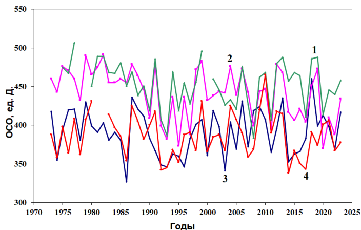
Рисунок 18.3 – Межгодовой ход средних за март значений ОСО на станциях: 1 – Нагаево (Магадан) (60° с.ш., 151° в.д.), 2 – Якутск (62° с.ш., 130° в.д.), 3 – С.-Петербург (60° с.ш., 30° в.д.) и 4 – Екатеринбург (57° с.ш., 61° в.д.)
