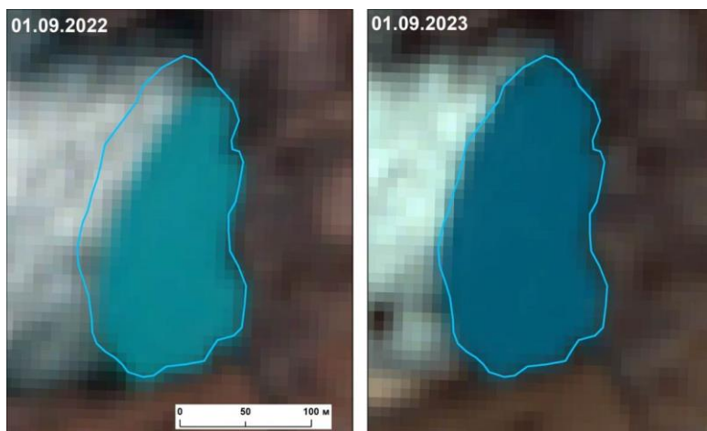
Рисунок 11.1 – Состояние озера Бирджалы Южное на севере Эльбруса в 2022 и 2023 гг.
