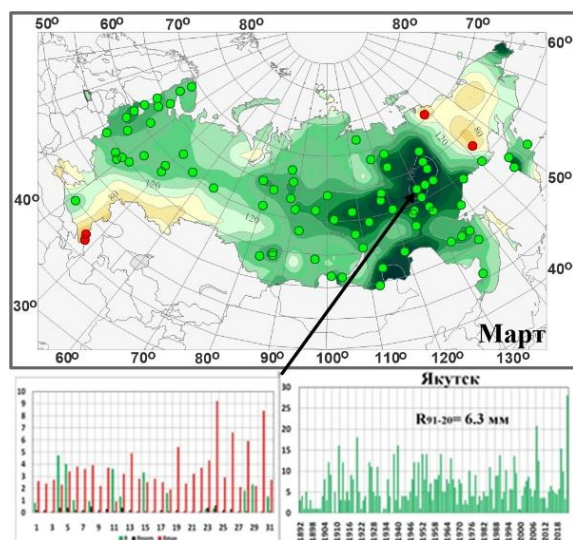
Рисунок 2.3 – Аномалии осадков в марте 2023 г. На врезках ряды месячных и суточных сумм осадков на метеорологической станции Якутск в зоне значительного переувлажнения
