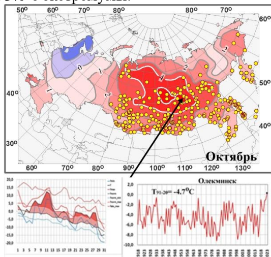
Рисунок 1.4 – Аномалии температуры приземного воздуха на территории России в октябре 2023. На врезках ряды среднемесячной октябрьской температуры воздуха и среднесуточной температуры воздуха в октябре 2023 года на метеорологической станции Олекминск в очаге максимальных температурных аномалий
