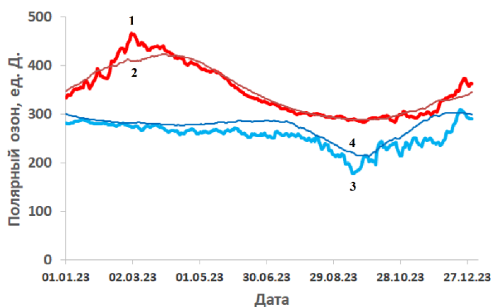
Рисунок 18.4 – Годовая изменчивость полярного озона в Арктике (1) и Антарктике (3) в 2023 г. Для сравнения представлен годовой ход средних многолетних значений полярного арктического (2) и антарктического (4) озона 1979-2022 гг.
