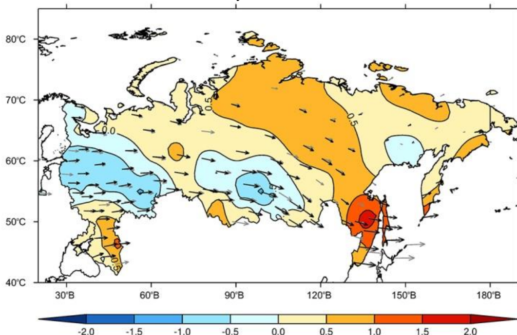
Рисунок 15.1 – Аномалии скорости ветра в 2023 г. в тропосфере. Черные стрелки указывают среднее направление ветра в 2023 г., серые – за период 1985-2014 гг.
