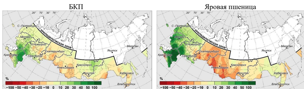
Рисунок 8.4 – Отклонения (%) значений биоклиматического потенциала и климатически обусловленной урожайности яровой пшеницы за 2023 г. относительно средних за 2018–2022 гг. Расчёты выполнены в имитационной системе Климат-Почва-Урожай
