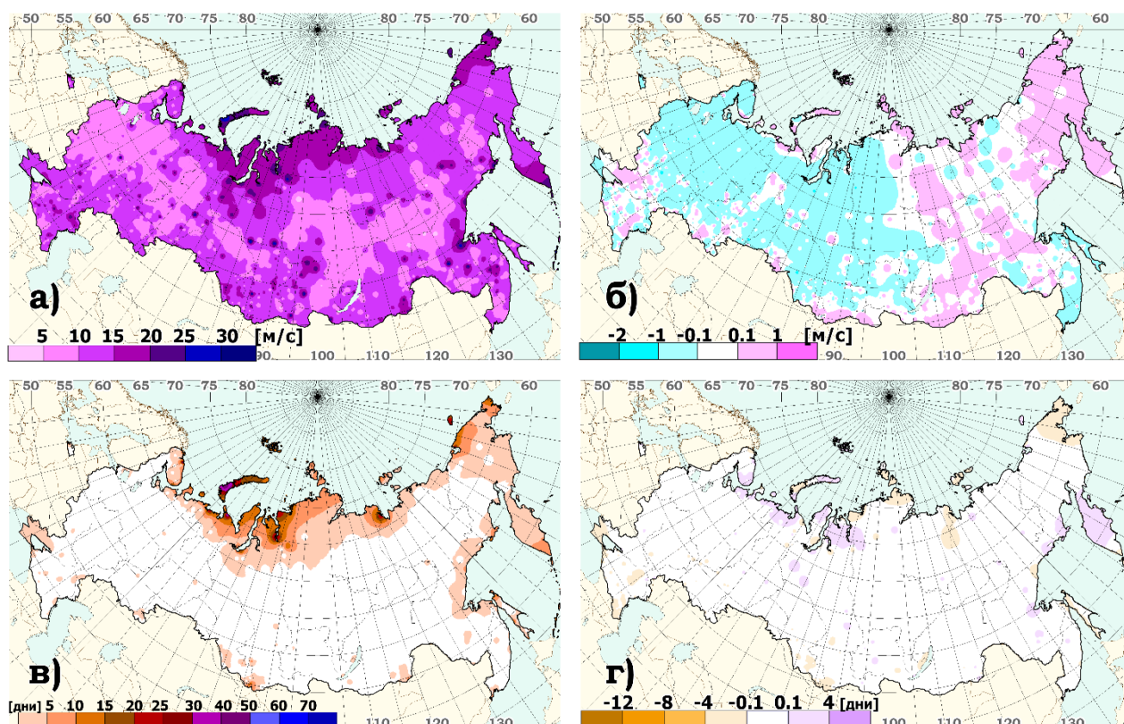
Рисунок 14.1 – а) Максимальная скорость ветра за 2023 г. (без учета порывов); б) Аномалии среднегодовой скорости ветра в 2022 г.; в) Число дней со скоростью ветра \geq 15 м/с в 2022 г.; г) Аномалии (отклонение от средних многолетних значений) числа дней со скоростью ветра \geq 15 м/с в 2023 г.
