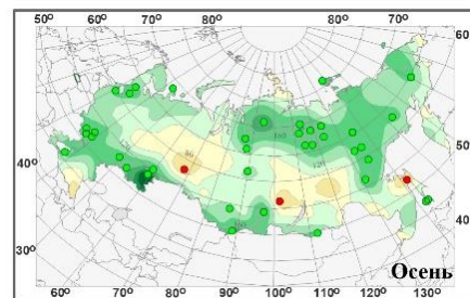
Рисунок 2.2 – Аномалии осадков на территории России в 2023 г., с указанием локализации 5%-х экстремумов (красные кружки) и 95%-х (зеленые кружки)
