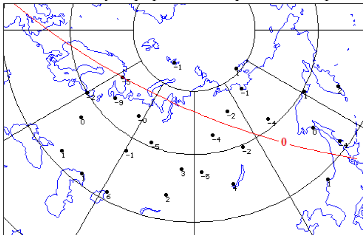
Рисунок 18.2 – Поле отклонений среднегодовых значений ОСО от средних многолетних значений в 2023 г., (%)
