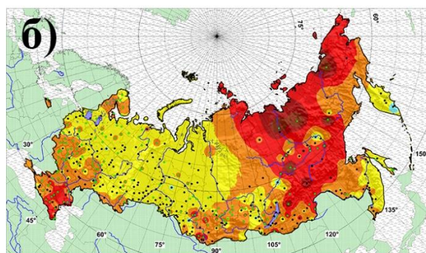
Рисунок 17.2 – Пространственное распределение трендов минимальной температуры почвы за 1976-2023 гг. на территории России ( ^{\circ}\text{C}/10 лет) на глубинах: а) 80 см, б) 160 см, в) 320 см. Точками показано расположение метеорологических станций со статистически значимыми (зеленые) и незначимыми (черные) коэффициентами линейного тренда
