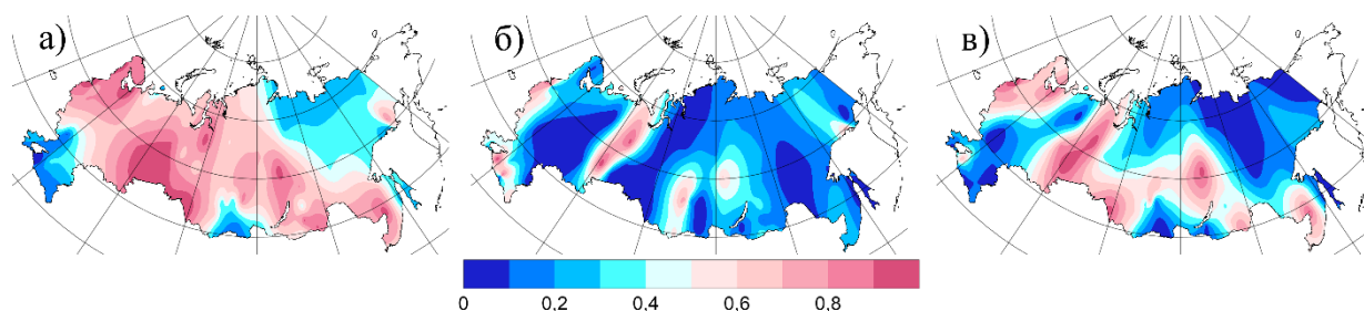
Рисунок 10.5 – Аномалии (в процентах от среднего за 1961-1990 гг.) сезонных сумм рассеянной (а) и суммарной (б) радиации. Весна 2023 г.
