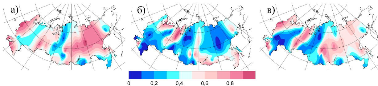
Рисунок 10.7 – Аномалии (в процентах от среднего за 1961-90 гг.) сезонных сумм рассеянной (а) и суммарной (б) радиации. Лето 2023 г
