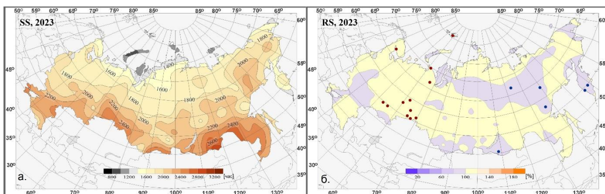
Рисунок 12.1 – Пространственное распределение суммарной за год продолжительности солнечного сияния (SS, часы) и ее относительных аномалий (RS, %) на территории РФ в 2023 г. (январь-декабрь). Кружками синего цвета показано местоположение станций с экстремумами ниже 5-го перцентиля, коричневого цвета – выше 95-го перцентиля
