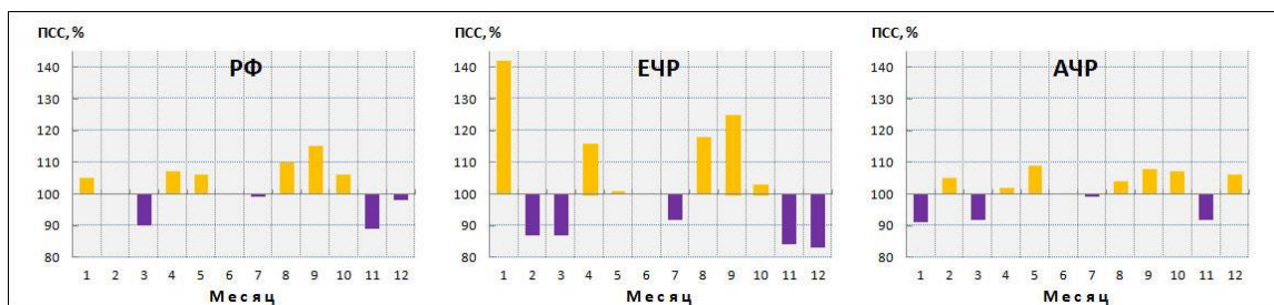
Рисунок 12.4 – Относительные аномалии суммарной за месяц продолжительности солнечного сияния, осредненной по территории РФ, ЕЧР и АЧР; 2023 г.
